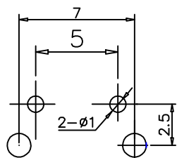
安装孔位图
